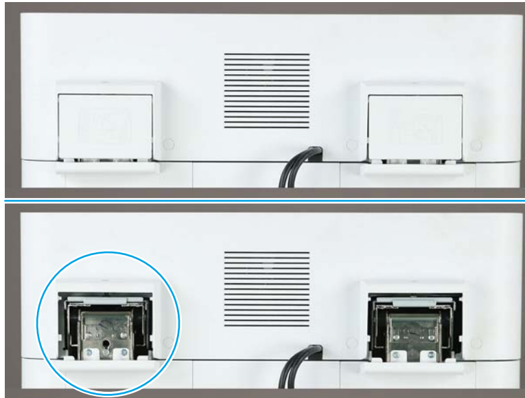
그림 7-12 ADF 힌지 조정
