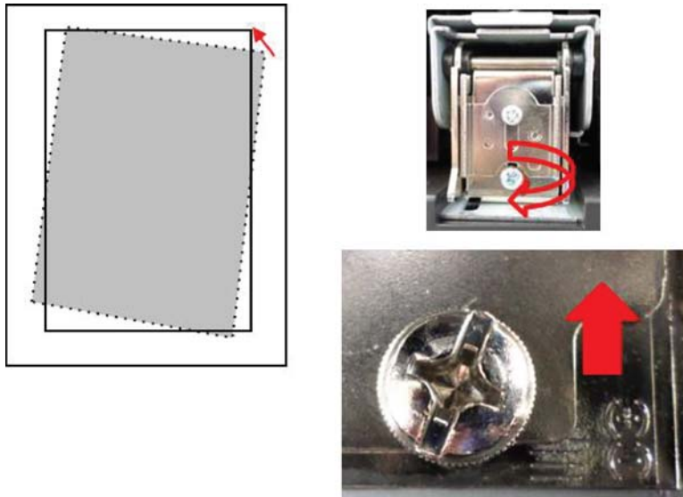
그림 7-14 힌지 조정
