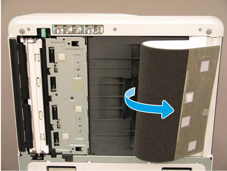
그림 7-8 ADF 장치 열기
