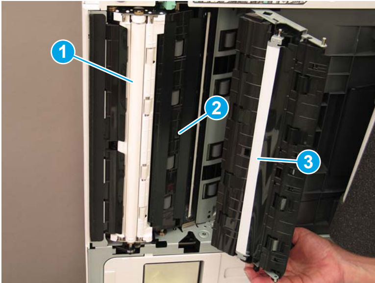
그림 7-9 ADF 흰색 막대 청소
