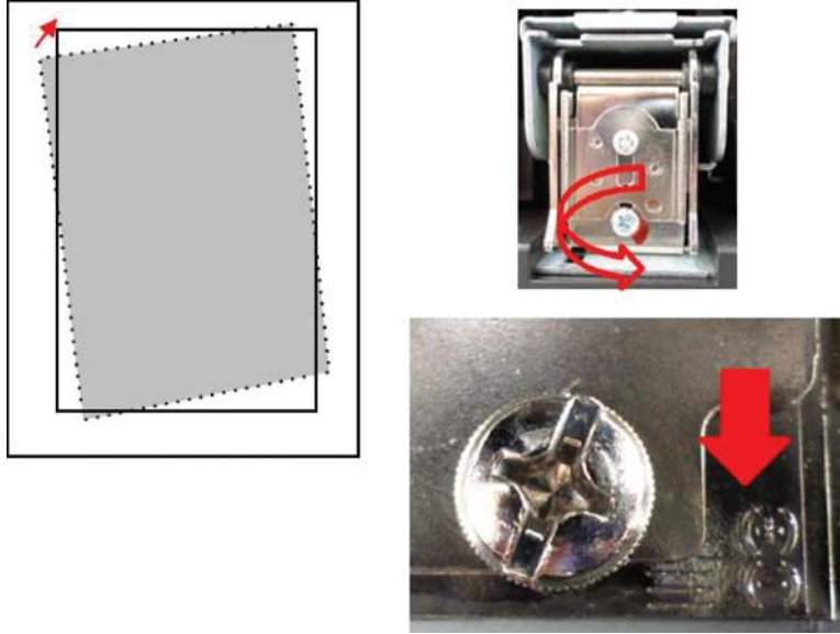
그림 7-13 힌지 조정
