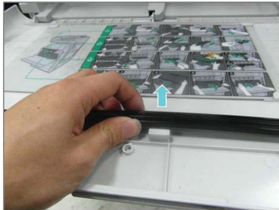
그림 7-4 레이저 스캐너 어셈블리 창 청소 도구를 제거합니다.
