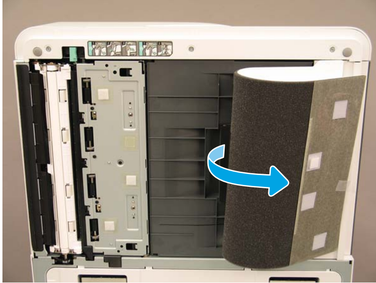
그림 7-6 ADF 장치 열기
