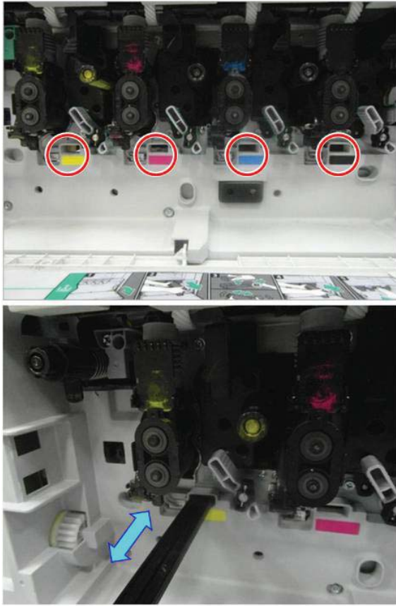
그림 7-5 레이저 스캐너 어셈블리 색상 입구
