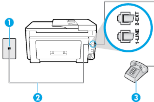
Abbildung 5-4 Rückansicht des Druckers
