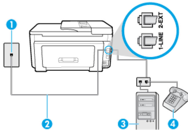
Abbildung 5-16 Rückansicht des Druckers
