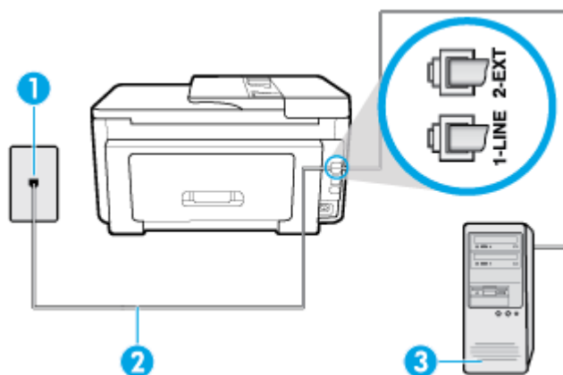
Abbildung 5-6 Rückansicht des Druckers
