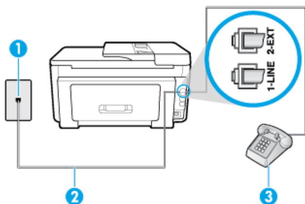
Εικόνα 5-4 Πίσω πλευρά εκτυπωτή
