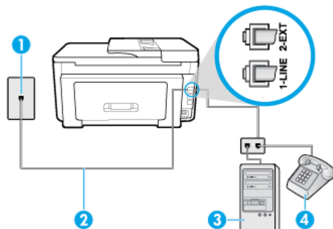
Εικόνα 5-16 Πίσω πλευρά εκτυπωτή
