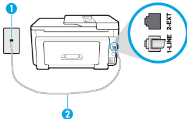
Εικόνα 5-5 Πίσω πλευρά εκτυπωτή
