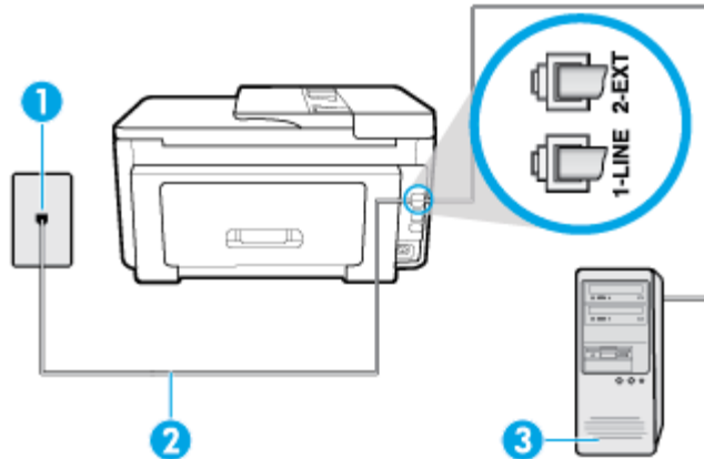
그림 5-6 프린터의 뒷 부분
