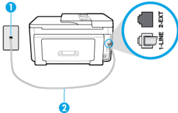
그림 5-5 프린터의 뒷 부분
