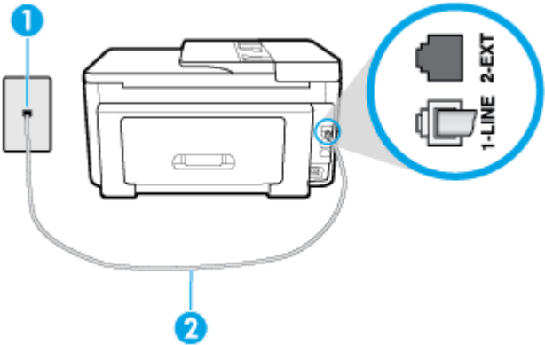
圖示 10-1 印表機的背視圖
