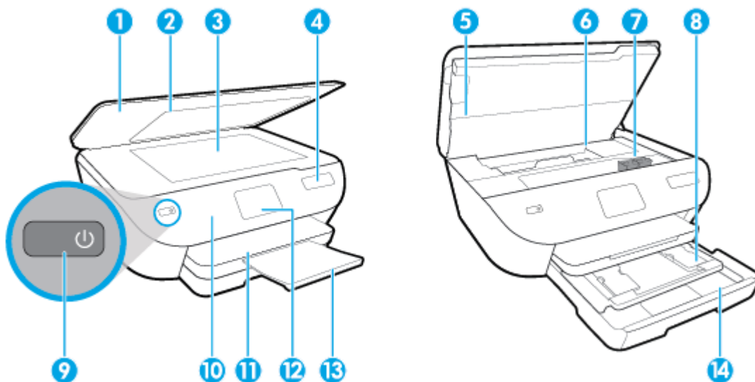
Hình 2-1 Mặt trước và trên của HP ENVY Photo 6200 All-in-One series
