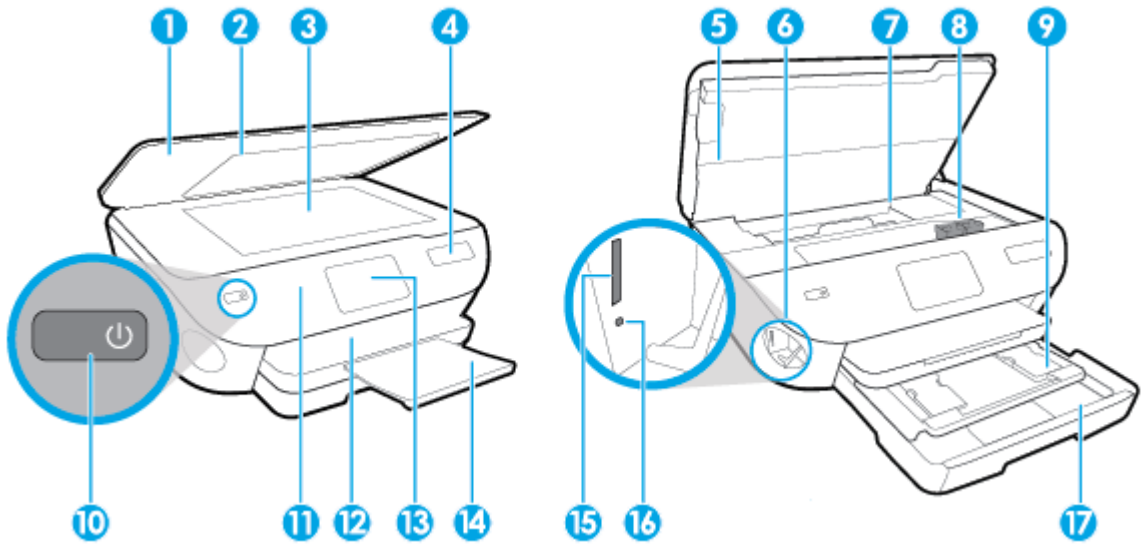
图 2-1 HP ENVY Photo 7100 All-in-One series 的前视图和上视图
