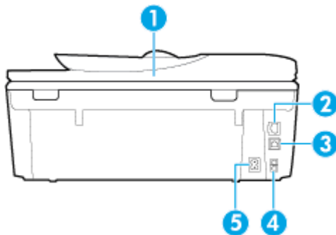
Figura 2-2 Vista posteriore di HP ENVY Photo 7800 All-in-One series
