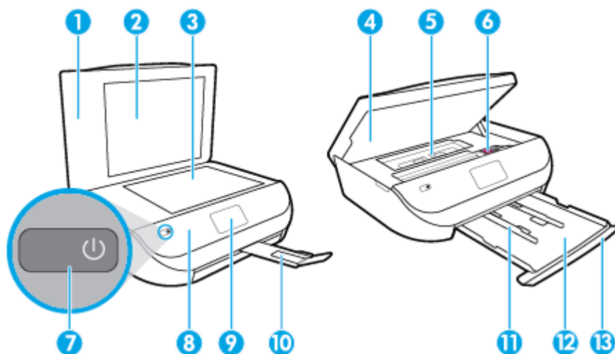
Joonis 2-1 Seadme HP DeskJet Ink Advantage 5000 All-in-One series eest- ja pealtvaade
