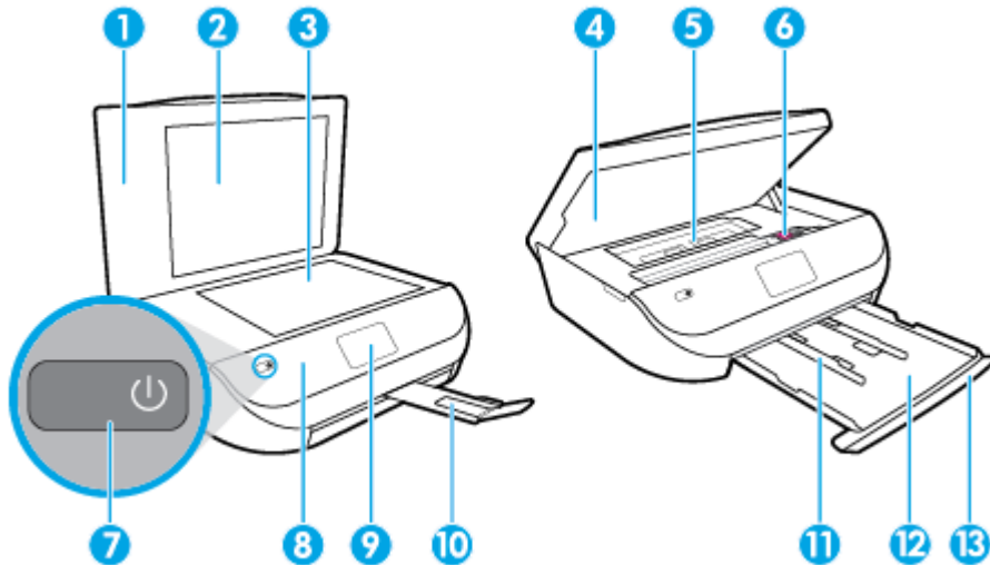
Kuva 2-1 HP DeskJet Ink Advantage 5000 All-in-One series edestä ja ylhäältä
