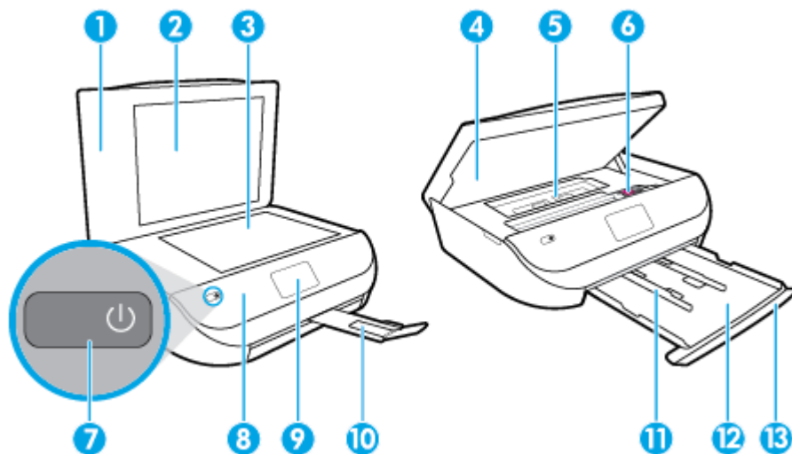
図 2-1 HP ENVY 5000 All-in-One series の正面および上面図
