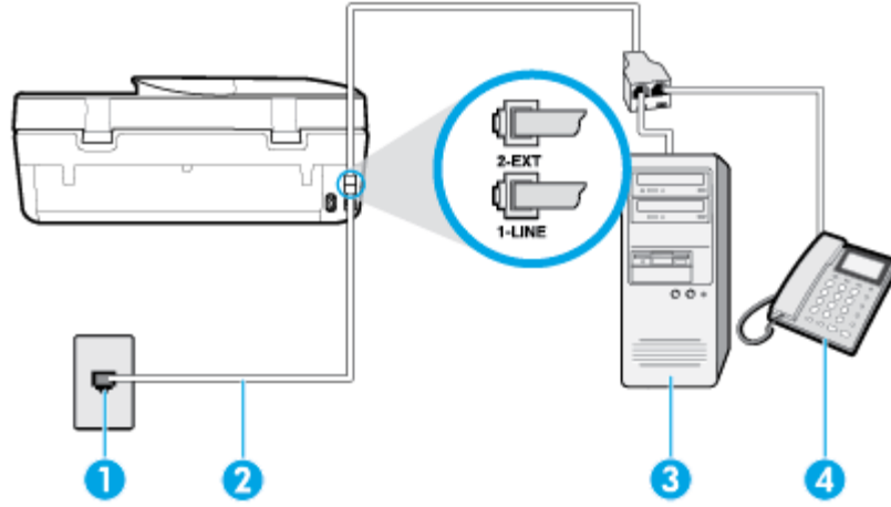
شكل ١٦-٥ منظر خلفي للطابعة
