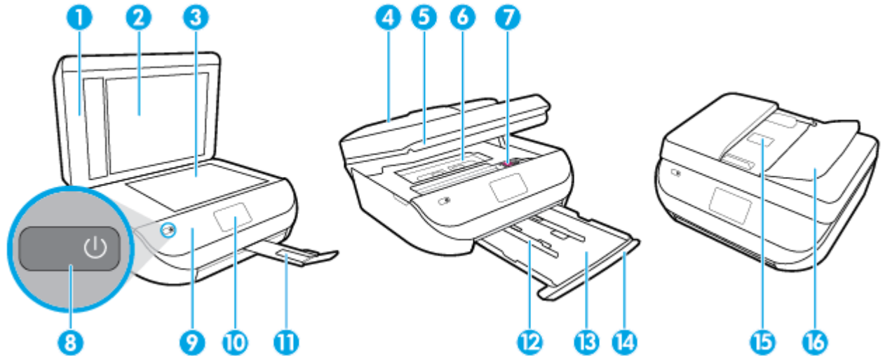
그림 2-1 HP DeskJet Ink Advantage 5200 All-in-One series의 앞면 및 윗면 뷰
