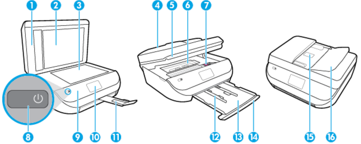
Şekil 2-1 HP DeskJet Ink Advantage 5200 All-in-One series ürününün önden ve üstten görünümü
