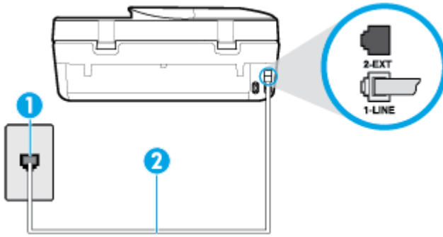
Şekil 5-5 Yazıcının arkadan görünümü
