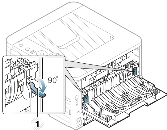
1 Druckhebel
