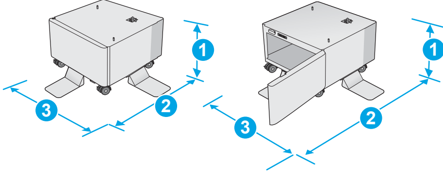
Şekil 1-3 Kabin/sehpa boyutları
