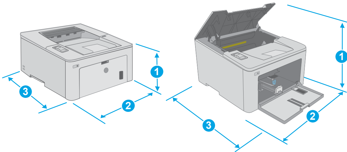
Εικόνα 1-1 Διαστάσεις του εκτυπωτή
