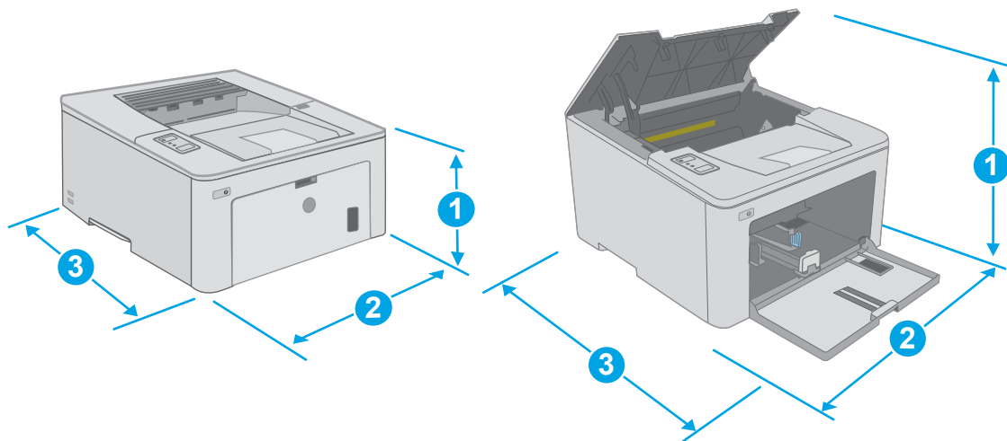
Рисунок 1-1 Розміри принтера
