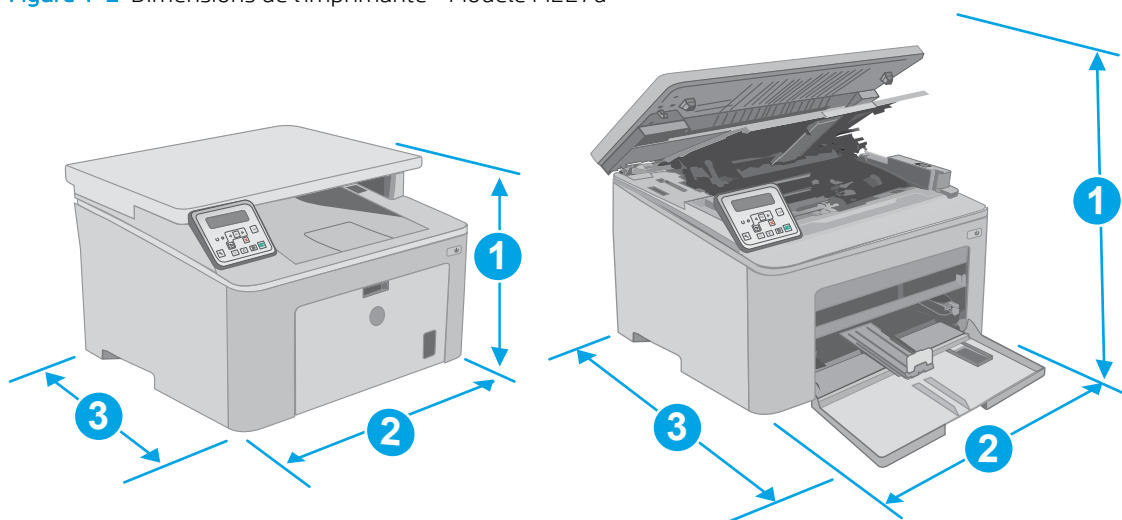
Figure 1-2 Dimensions de l'imprimante - Modèle M227d
