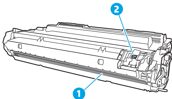
Bild 3-1 Tonerkassettdelar
