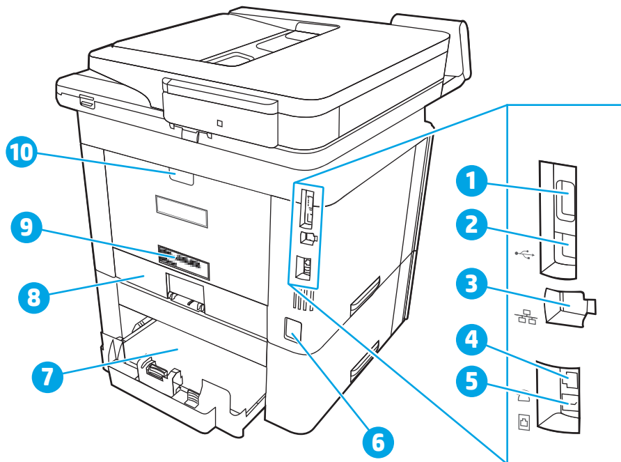
Bild 1-2 Skrivarens baksida
