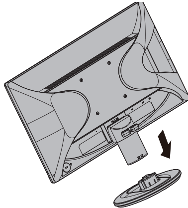
Figura 3-4 Extracción de la base del monitor
