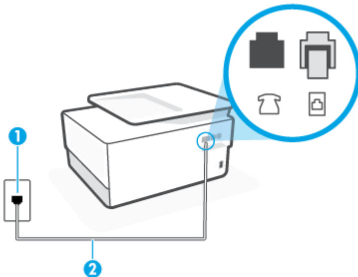
図 4-3 プリンターの背面図
