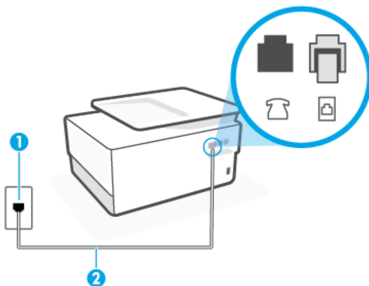
図 9-1 プリンターの背面図
