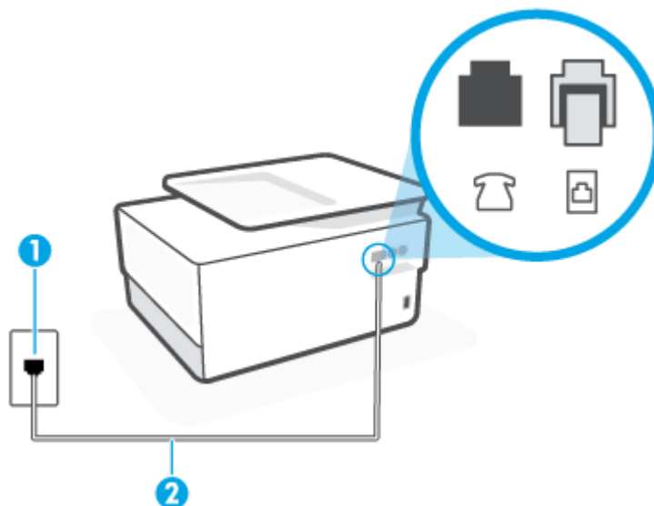
図 4-1 プリンターの背面図
