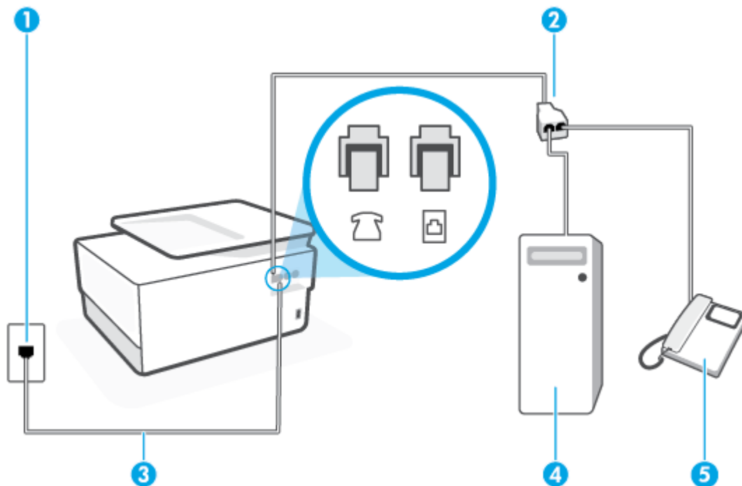
Figura 4-9 Vedere din spate a imprimantei
