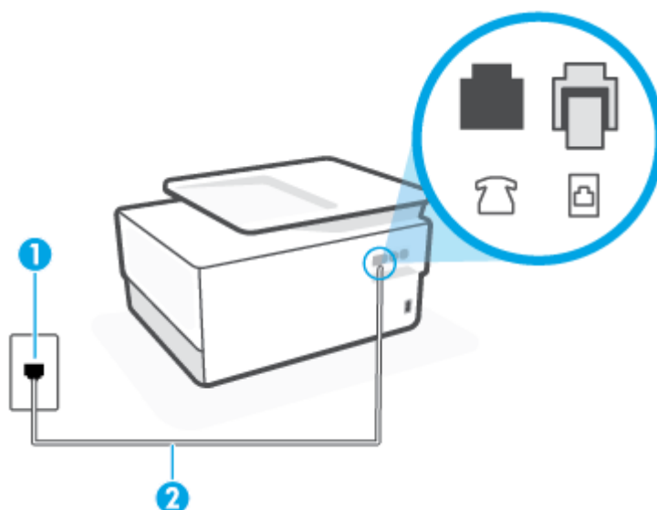
Figura 4-1 Vista posterior de la impresora
