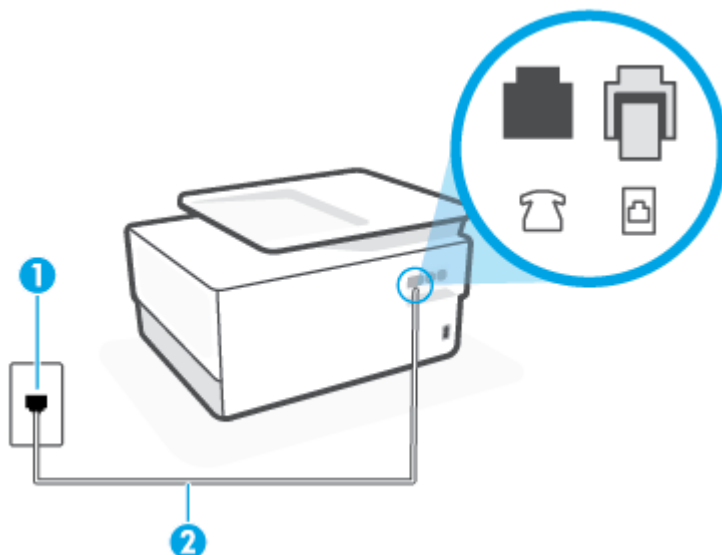
Figura 4-3 Vista posterior de la impresora
