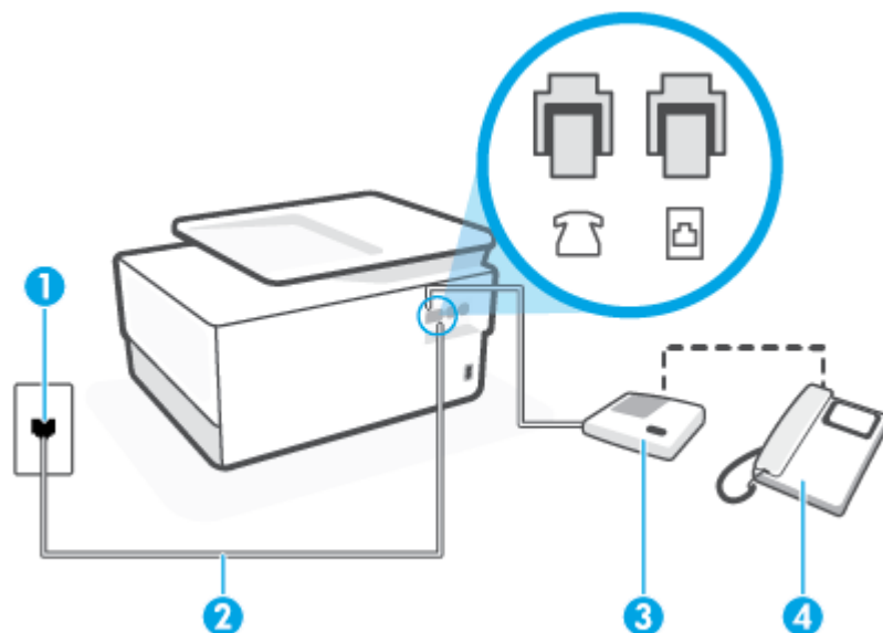
Figura 4-11 Vista posterior de la impresora
