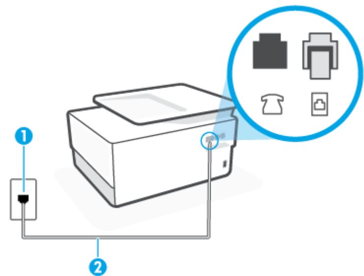
Figura 4-5 Vista posterior de la impresora
