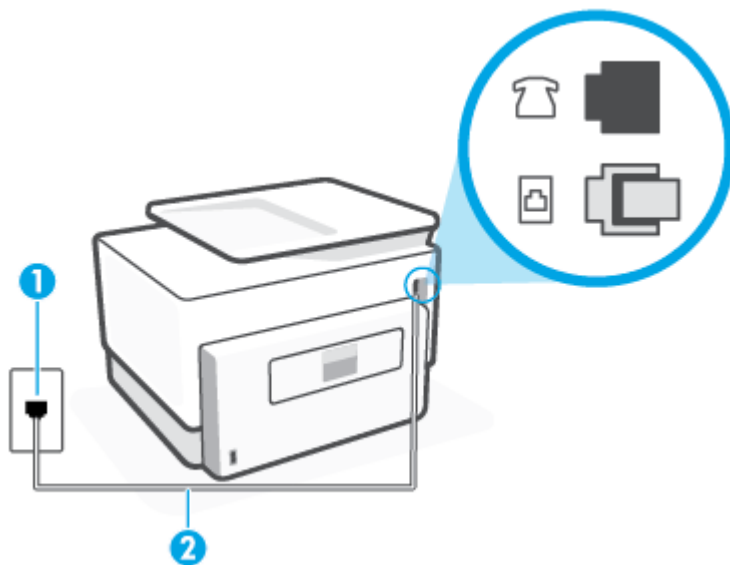
Фигура 4-5 Изглед на принтера отзад
