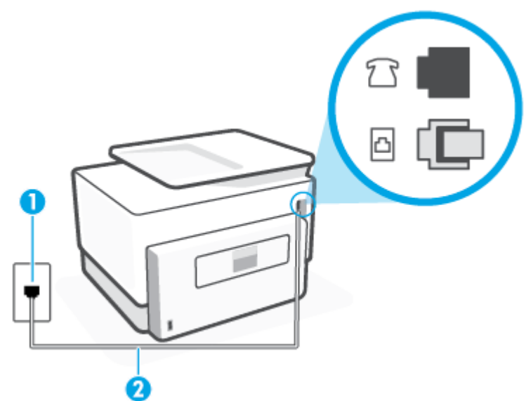
Figura 4-3 Vista posterior de la impresora
