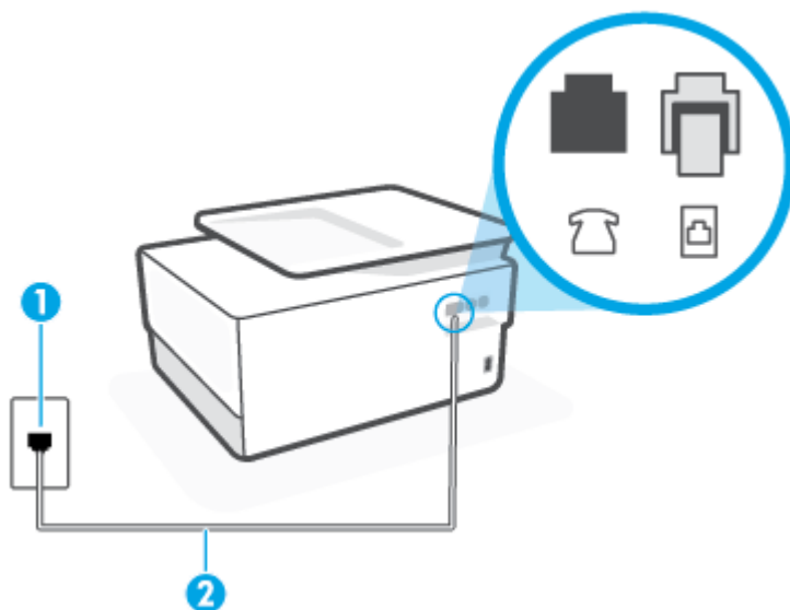
Figura 9-1 Vista posterior da impressora
