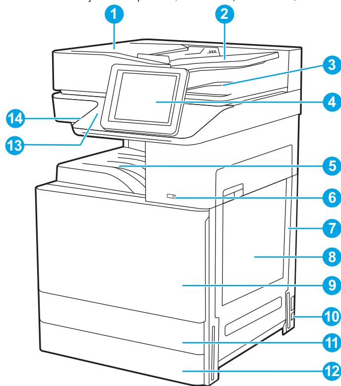
Slika 1-1 Prednja strana pisača (E72430dn, E72425dn)
