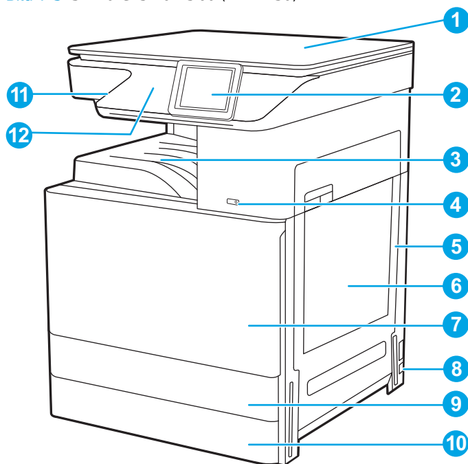
Bild 1-3 Skrivarens framsida (E72425a)
