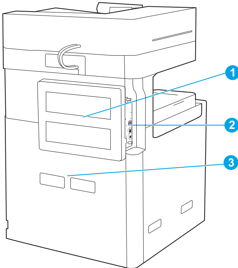
Bild 1-4 Skrivarens baksida
