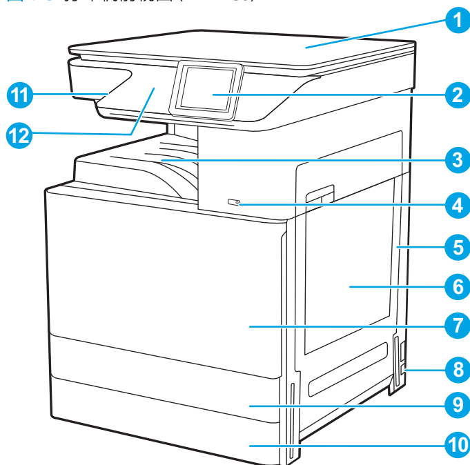
图 1-3 打印机前视图 (E72425a)
