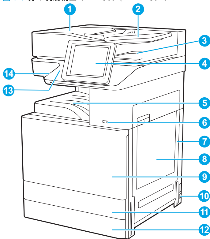
图 1-1 打印机前视图 (E72430dn、E72425dn)
