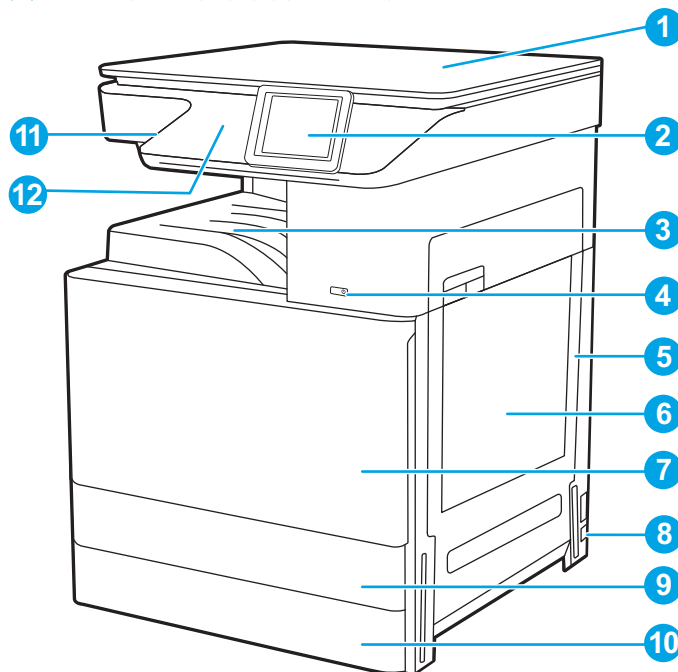
圖示 1-3 印表機前視圖 (E72425a)
