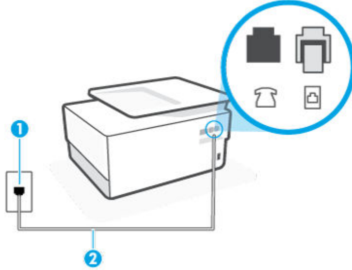
شكل ٩-١ المنظر الخلفي للطابعة
