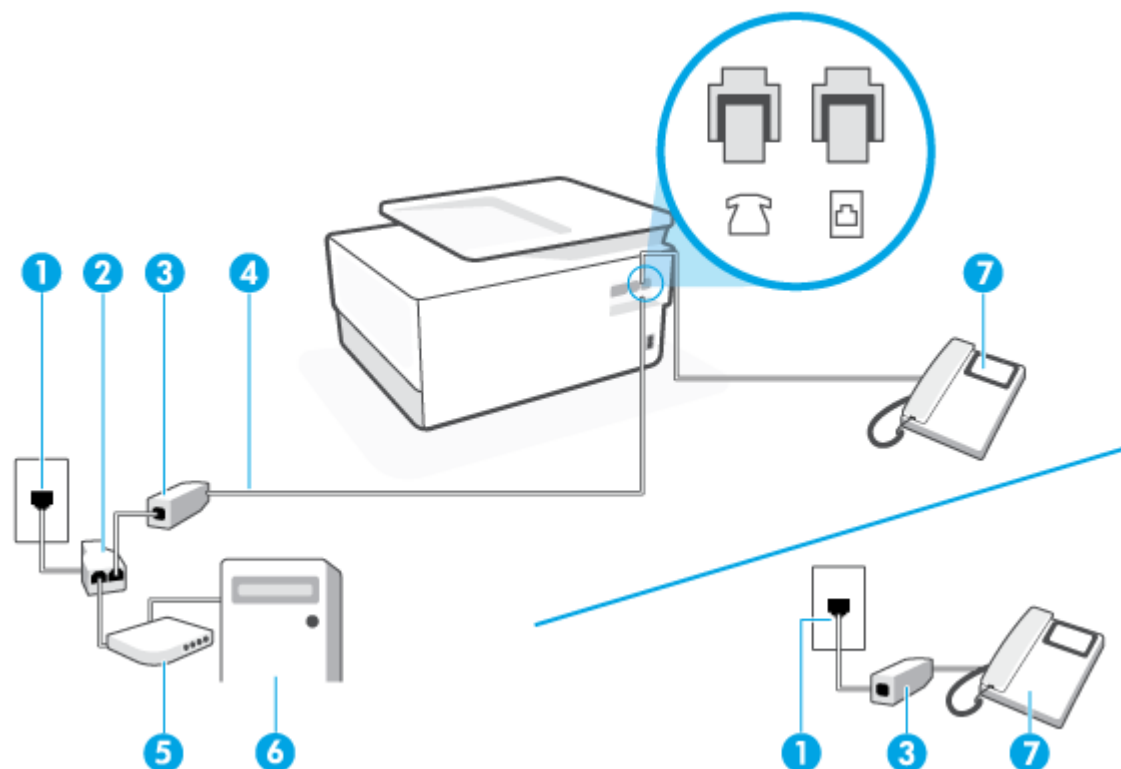
Εικόνα 4-10 Πίσω πλευρά εκτυπωτή
