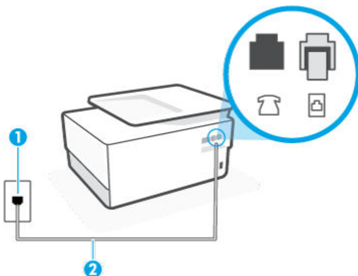
4-1. ábra: A nyomtató hátoldala
