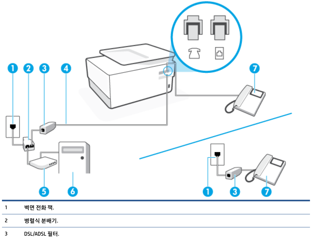
그림 4-10 프린터 뒷면
