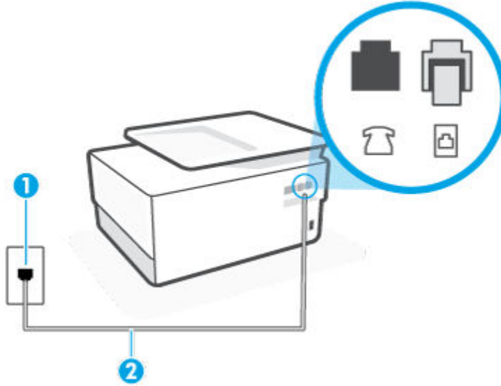
그림 9-2 프린터 뒷면
