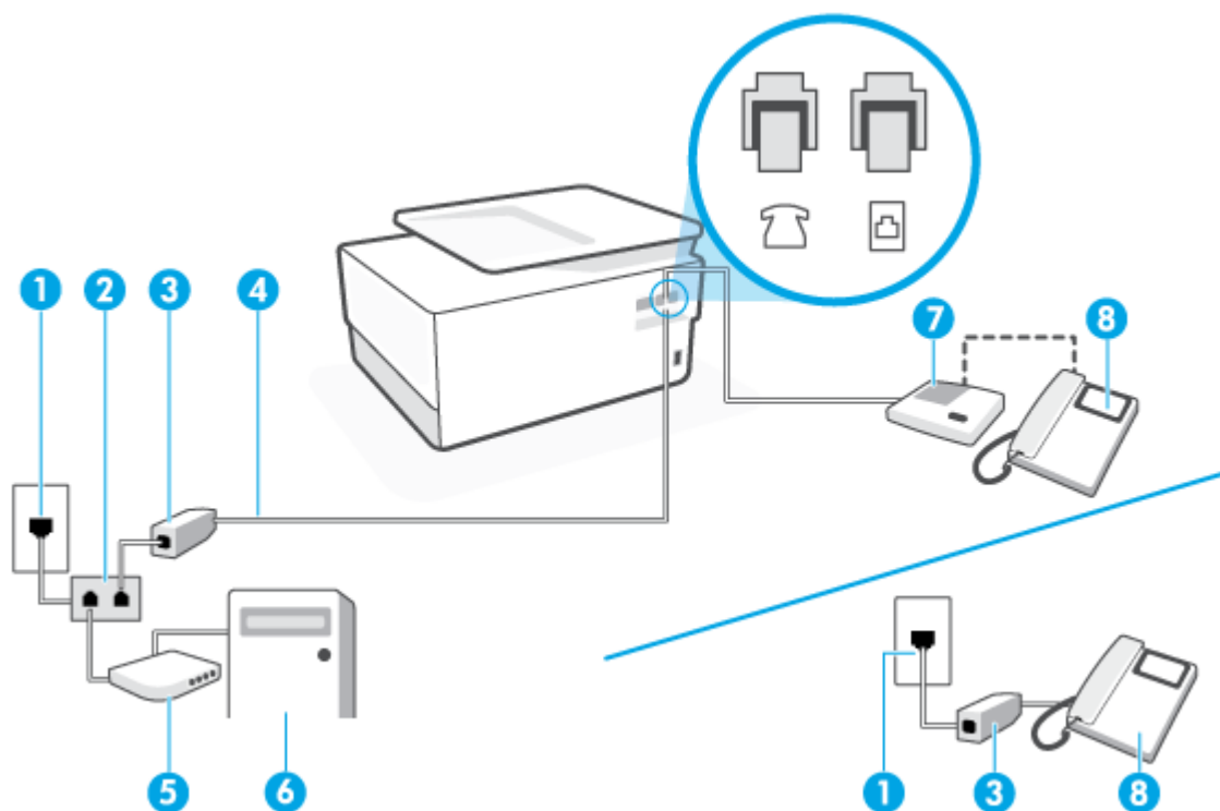
Figura 4-14 Vista posterior de la impresora
