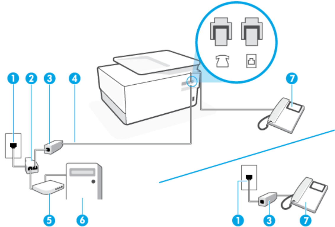
Figura 4-10 Vista posterior de la impresora
