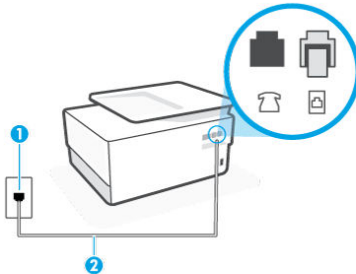
Figura 4-5 Vista posterior de la impresora
