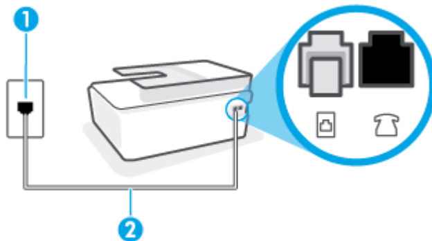
Εικόνα 5-3 Πίσω πλευρά εκτυπωτή
