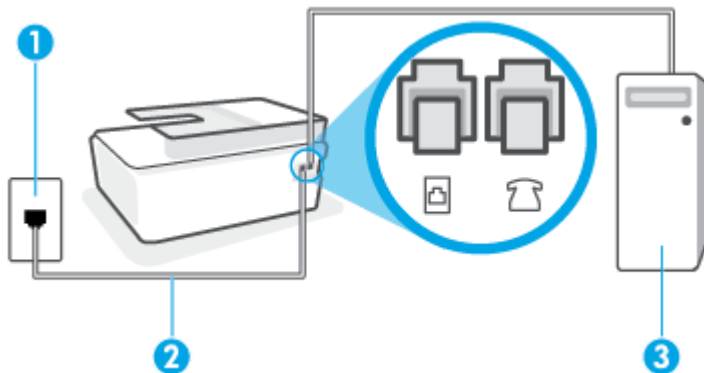
그림 5-6 프린터의 뒷 부분
