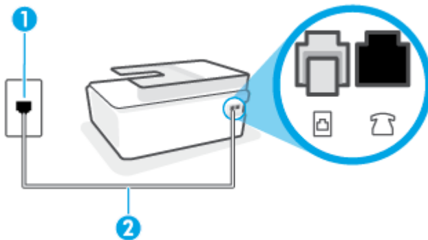
그림 5-5 프린터의 뒷 부분
