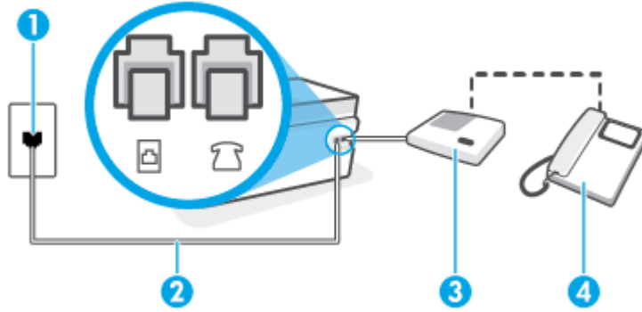
그림 5-11 프린터의 뒷 부분
