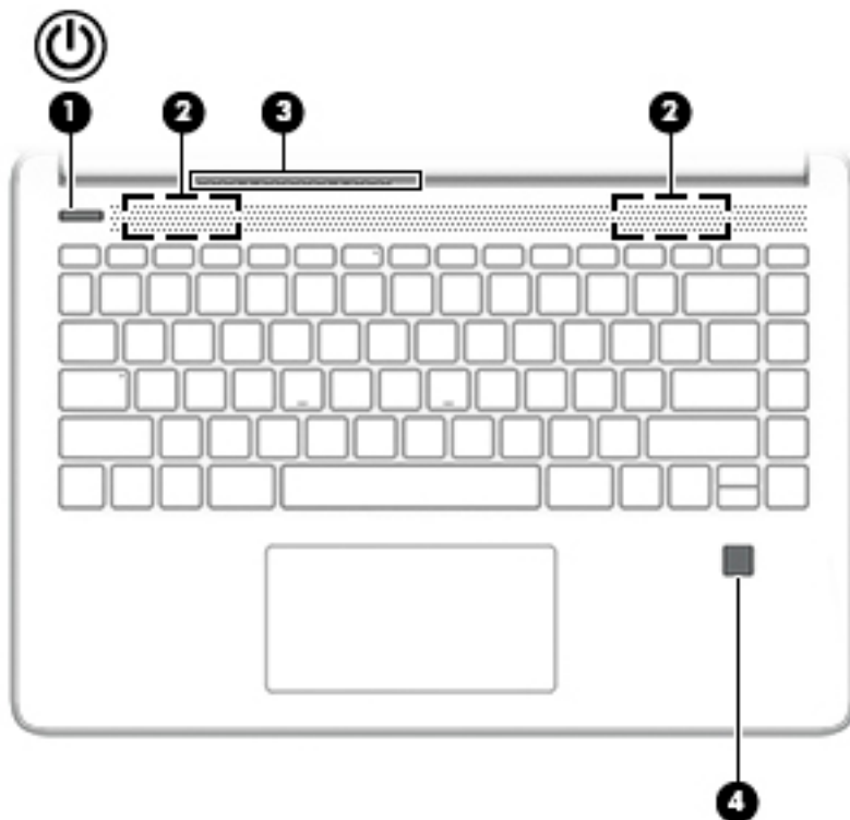
Кесте 2-6 Түйме, желдеткіш саңылау, үндеткіштер және саусақ ізін оқу құрылғысы және олардың сипаттамалары
