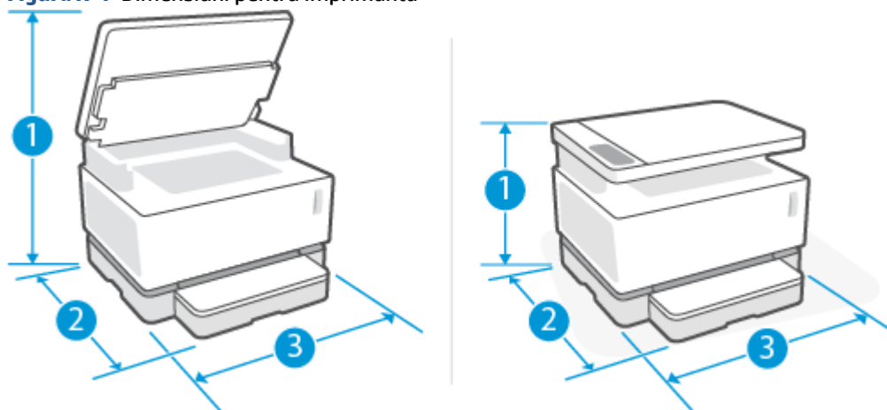
Figura A-1 Dimensiuni pentru imprimantă
