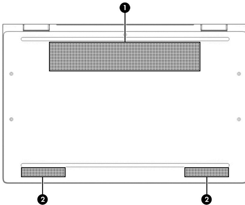
Tabuľka 2-11 Súčasti na spodnej strane a ich popisy
