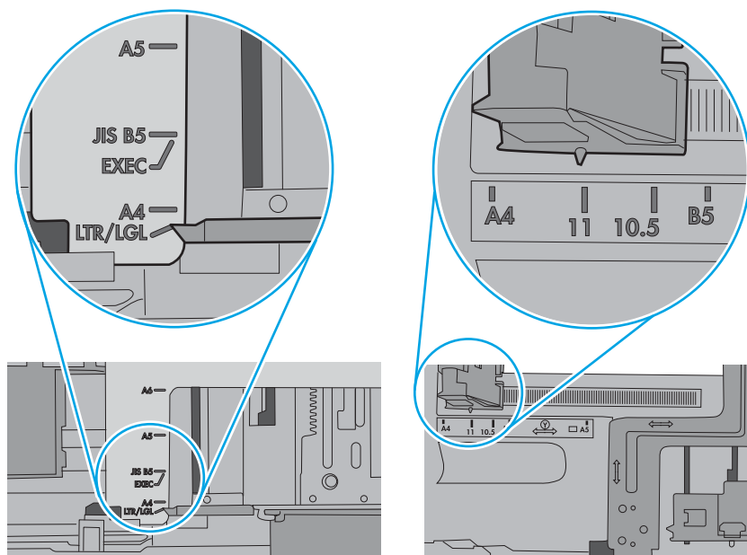
Сурет 9-9 Кассета науаларына арналған өлшем белгілері
