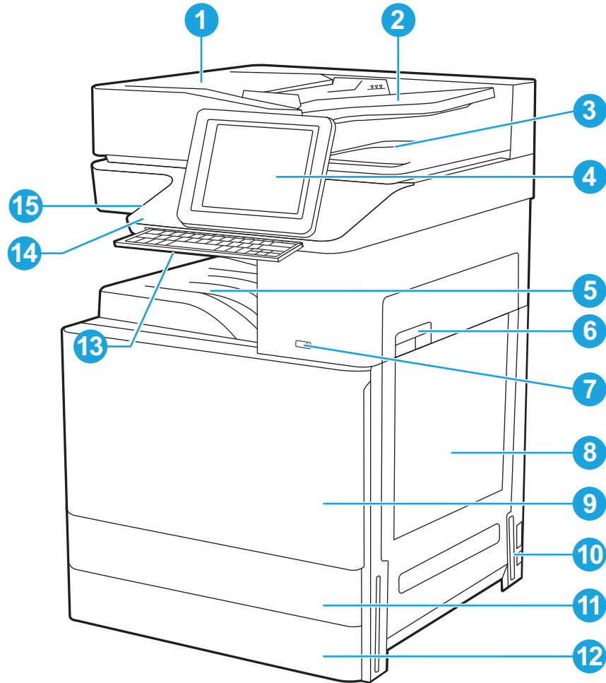
Сурет 1-1 Принтердің алдыңғы көрінісі
