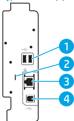
Сурет 1-3 Интерфейстік порттар көрінісі
