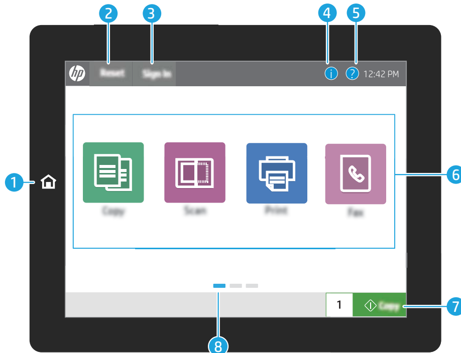
그림 1-4 제어판 보기
