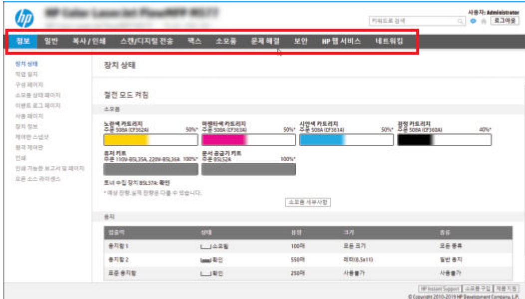
그림 8-1 EWS 탭
