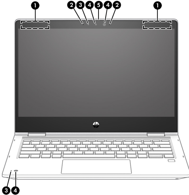
جدول ٣-٢ مكونات شاشة العرض ومواصفاتها
