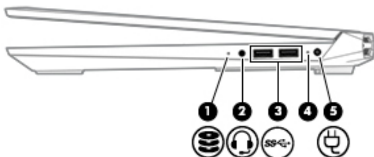
2-1 lentelė Dešinės pusės komponentai ir jų aprašymas
