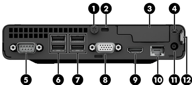
2-4 lentelė Supažindinimas su galinio skydelio komponentais
