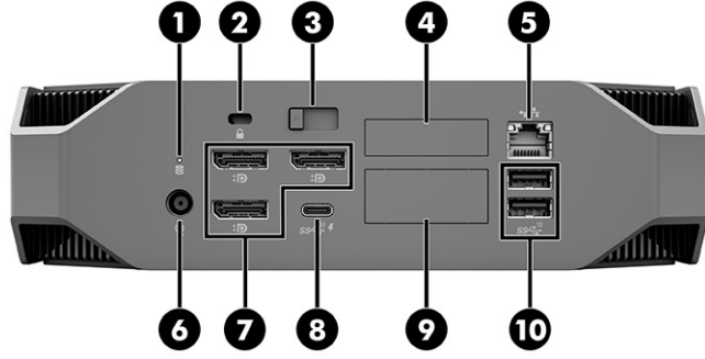
جدول ٢-٢ مكوّنات الجهة الخلفية ومواصفاتها
