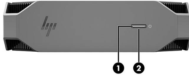
جدول ١-٢ مكونات الجهة الأمامية ومواصفاتها
