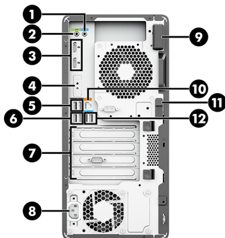
Πίνακας 2-4 Τα στοιχεία της πίσω πλευράς σε κατακόρυφο προσανατολισμό και οι περιγραφές τους
