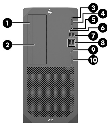
Πίνακας 2-3 Τα στοιχεία της πρόσοψης σε κατακόρυφο προσανατολισμό και οι περιγραφές τους
