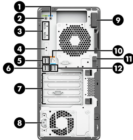
Таблиця 2-4 Компоненти задньої панелі башти та їхній опис
