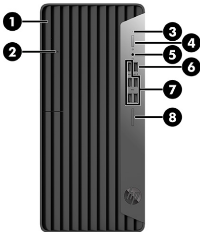
Таблиця 2-2 Визначення компонентів передньої панелі
